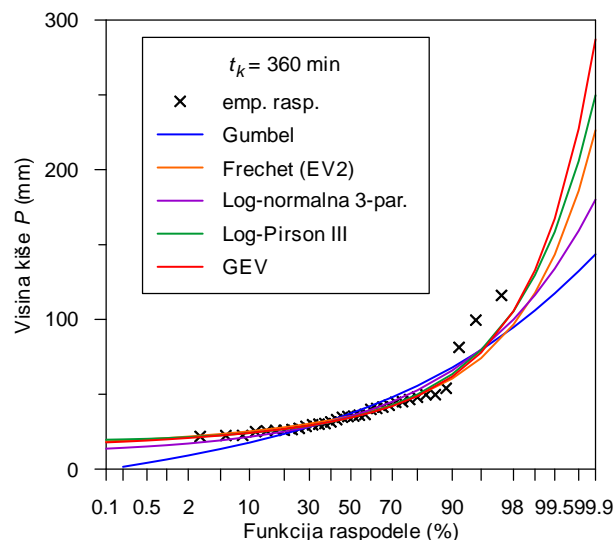
Slika 1. Raspodele verovatnoće visine kiše trajanja 360 minuta u Banja Luci prema različitim teorijskim raspodelama.
