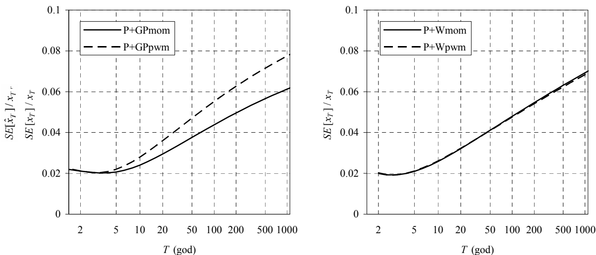
Slika 5. Relativna standardna greška ocene kvantila za dve metode ocene parametara na stanici Bezdán na Dunavu u modelima P+GP (levo) i P+W (desno); mom: metoda momenata; pwm: metoda težinskih momenata.
