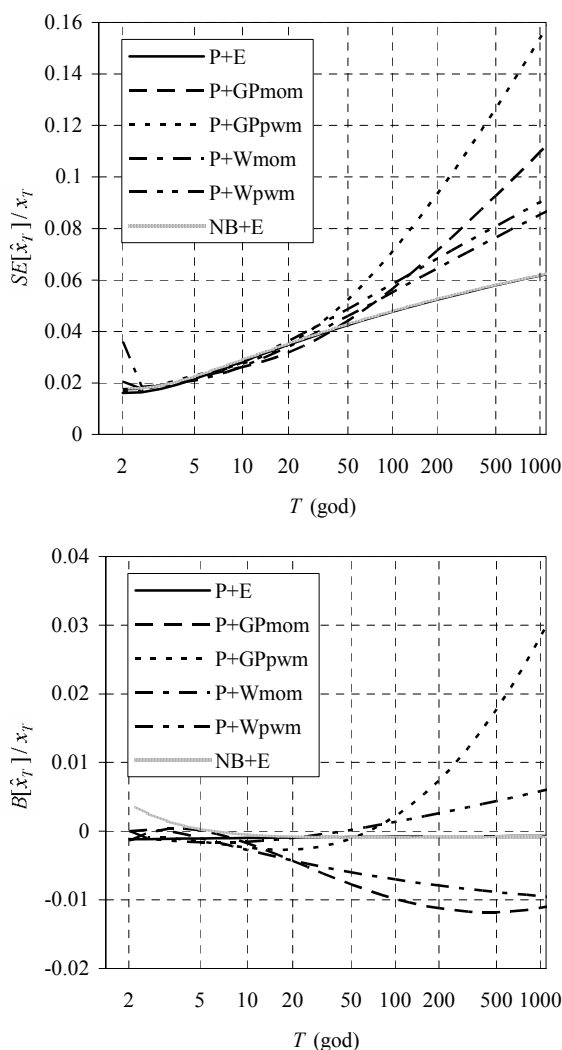
Slika 7. Relativna standardna greška (gore) i relativna pristrasnost (dole) ocene kvantila prema različitim modelima parcijalnih serija za stanicu Bezdan na Dunavu za bazu od 5000 m 3 /s.
