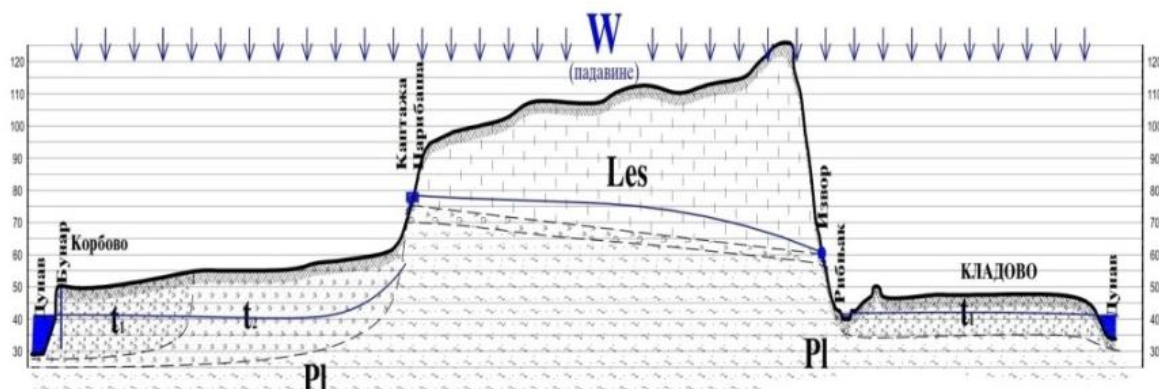
Slika 4. Geološki profil terena Korbovo-Kladovo [1]
