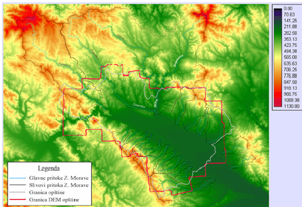
Slika 2. DMT opštine i slivnog područja pritoka reke Zapadne Morave (koja nije prikazana na slici) [11]
