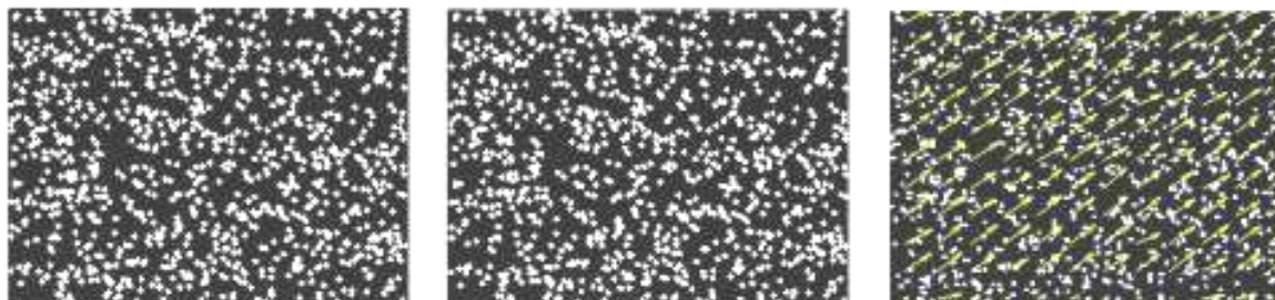
Slika 6: Testiranje softvera 1
