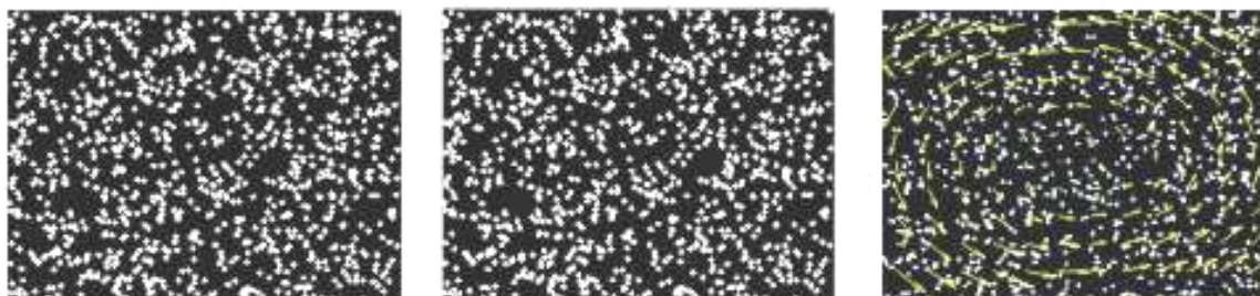
Slika 7: Testiranje softvera 2
